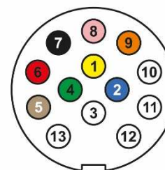
prise 13 broches
